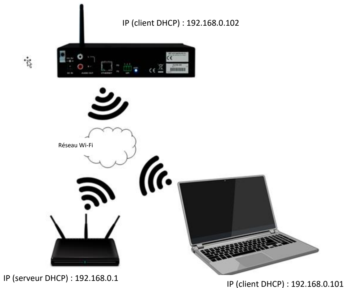
Figure 12 : exemple de connexion à un réseau local par l'interface réseau Wi-Fi (sans fil).
