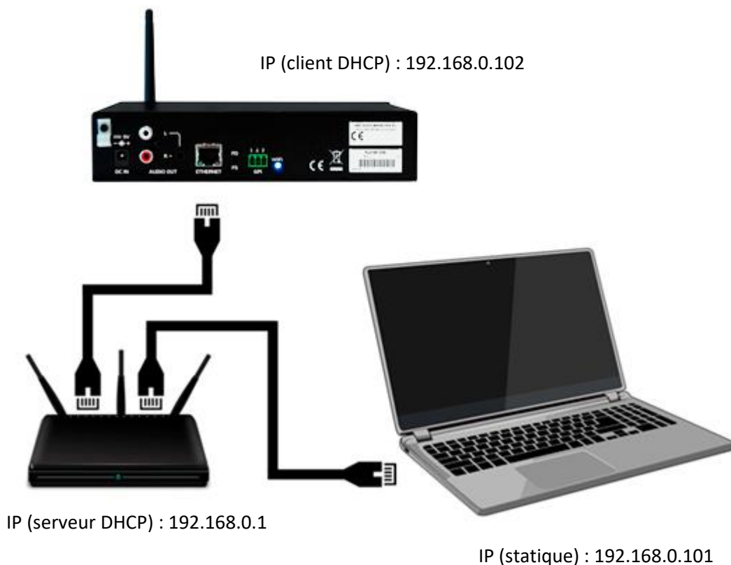
Figure 11 : exemple de connexion à un réseau local par l'interface réseau Ethernet (filaire).
