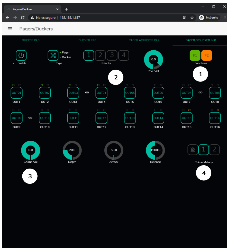
Abbildung 44: Seite zur Konfiguration eines Pagers
