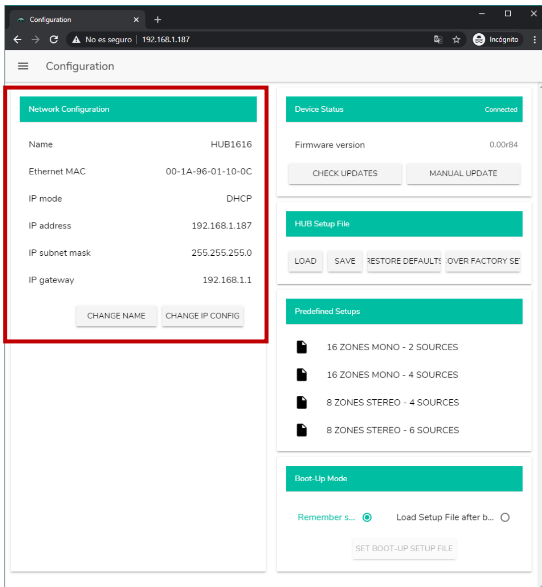
Abbildung 8: Netzwerk-Konfiguration
