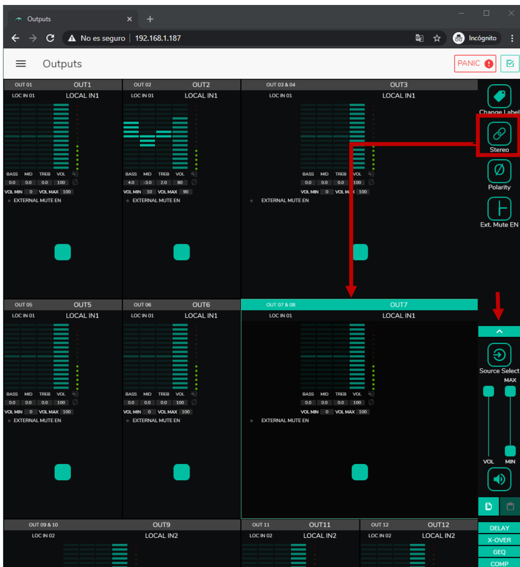
Figure 35 : sorties configurées en paire stéréo
