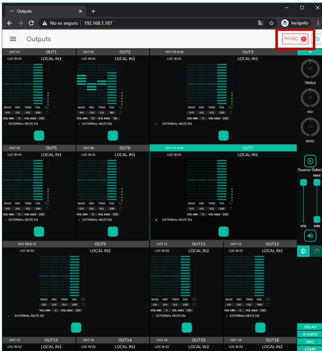
Figure 41 : bouton PANIC pour HUB1616
