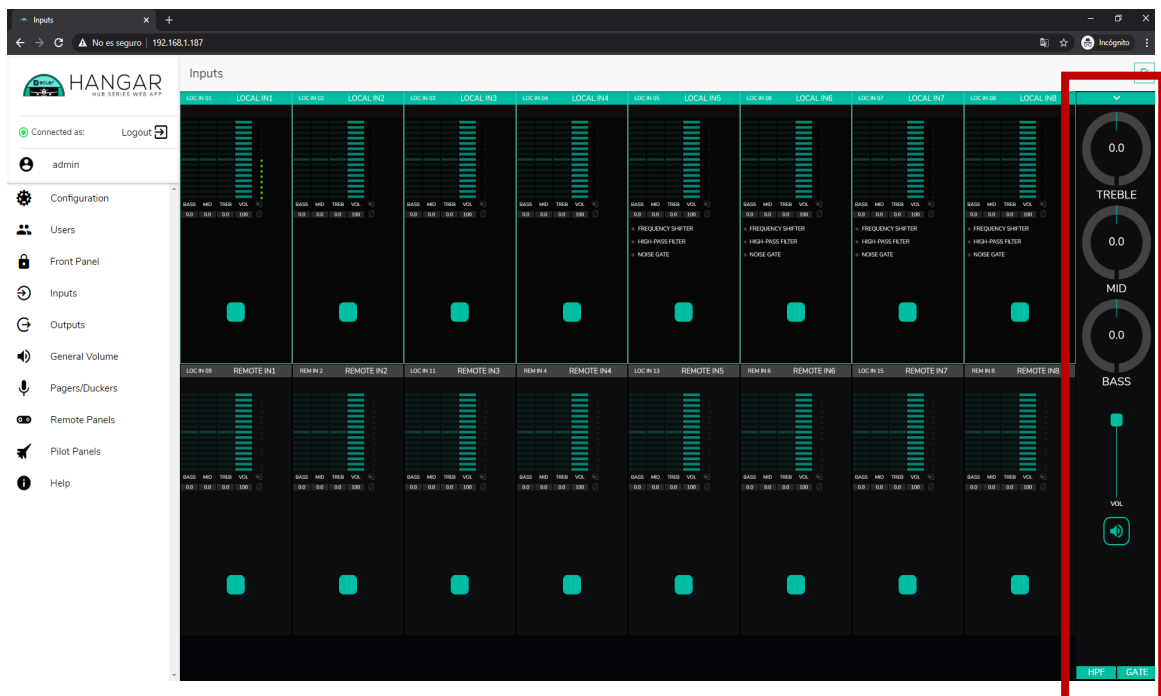
Figure 24 : contrôle et paramétrage des entrées
