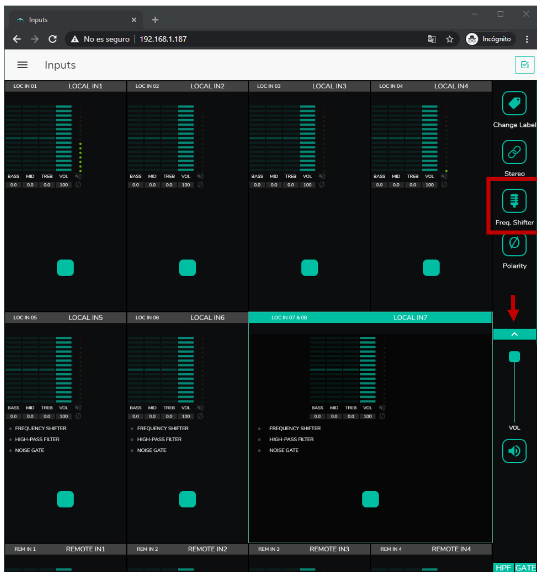
Figure 28 : activation du supprimeur de rétroaction (FREQUENCY SHIFTER)
