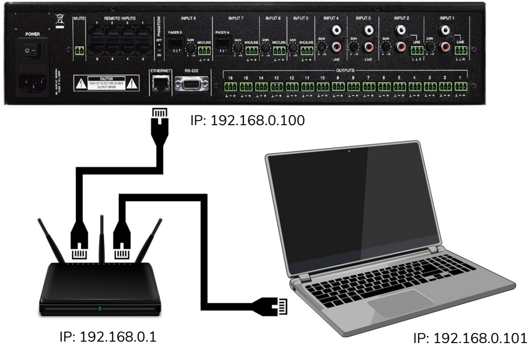
Figure 3 : connexion au réseau local (LAN)
