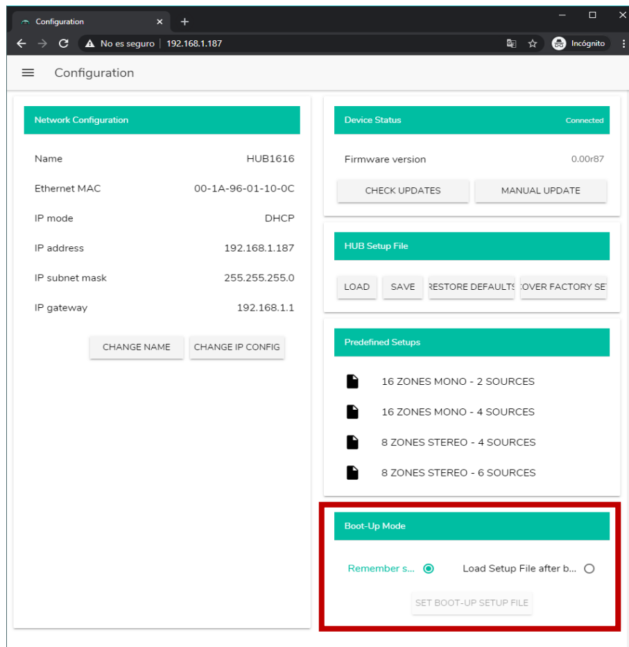
Figure 12 : configuration du mode de démarrage
