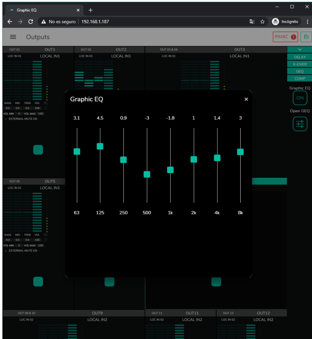
Figure 39 : réglage de l'égaliseur graphique sur une sortie
