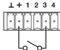
Ejemplo de conexionado del GPI 3
