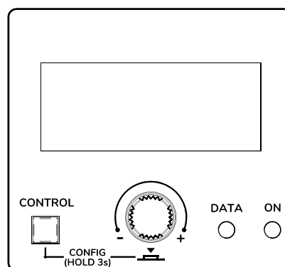
Figura 16: pantalla LCD del panel frontal y teclas de control
