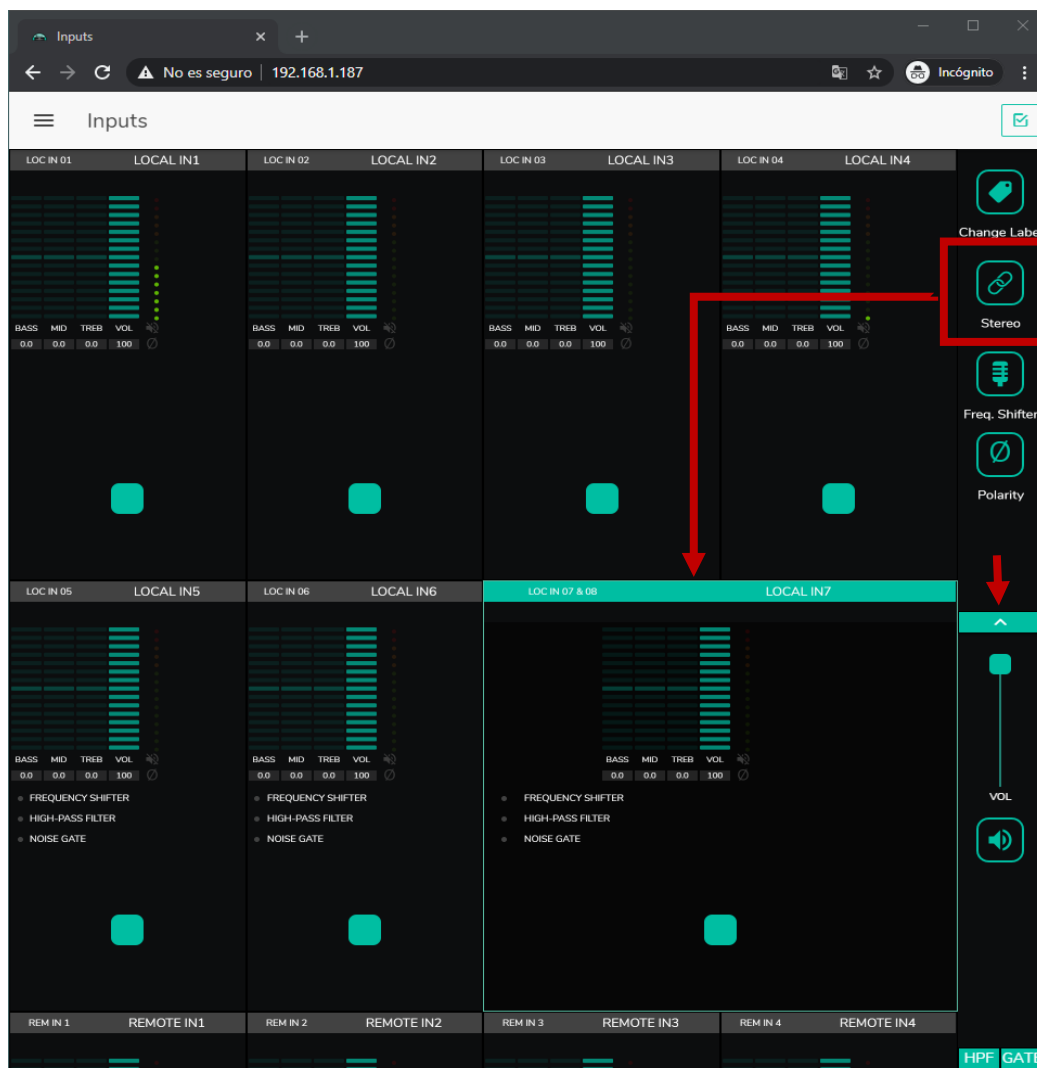
Figura 42: conversión de 2 entradas mono a estéreo
