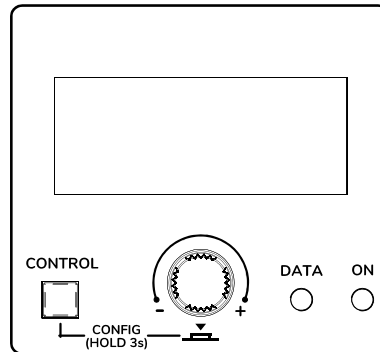
Figura 14: pantalla LCD del panel frontal y teclas de control
