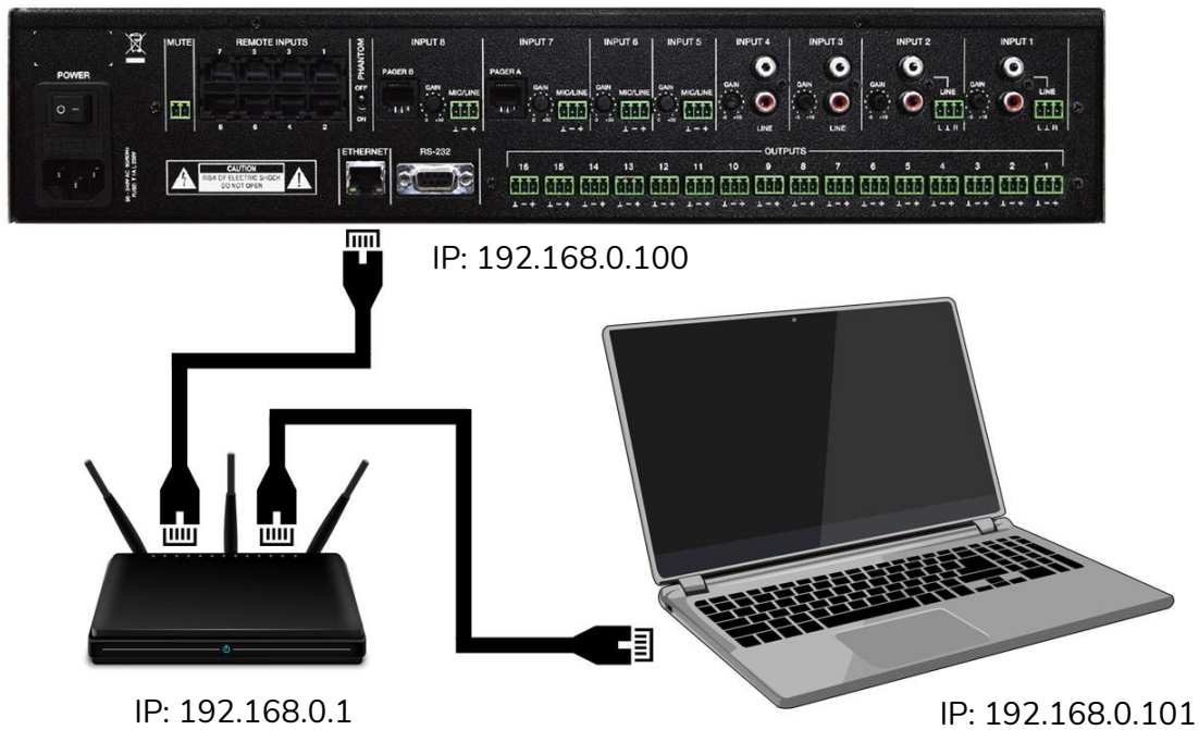
Figura 18: conexión en red local LAN
