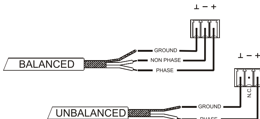
Figura 10: conexión de salida de audio balanceada
