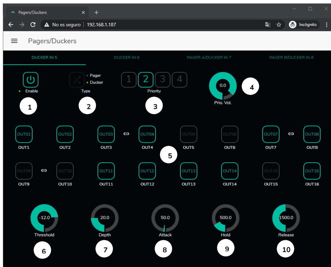
Figura 58:página pagers/duckersZZ
