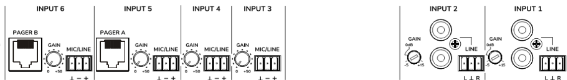
Abbildung 2: lokale Eingänge HUB1408
