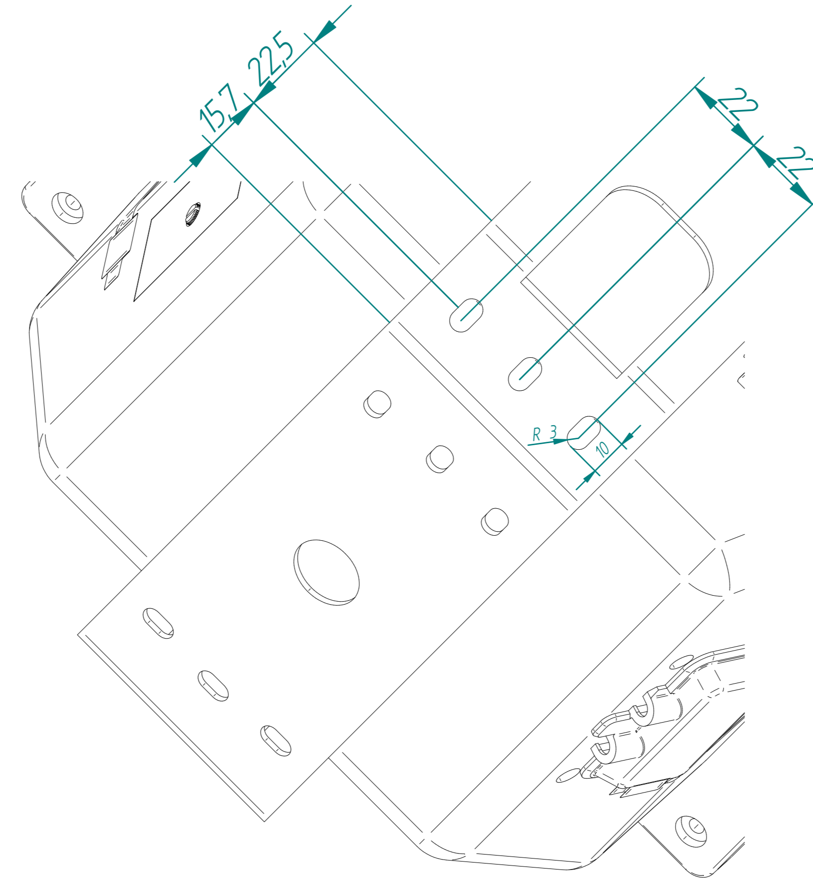
VISTA A
