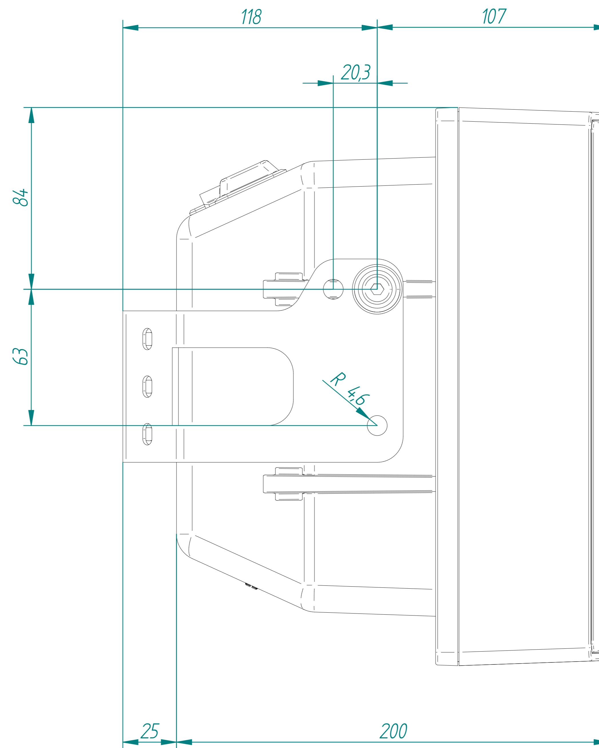
VISTA A
