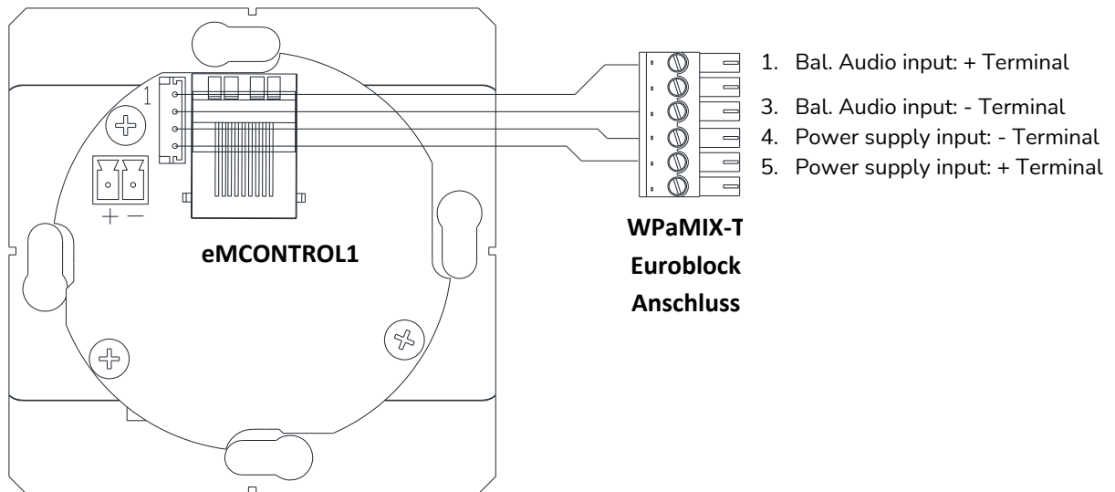
Abbildung 1: Anschlussdiagramm eMCONTROL1 + WPaMIX-T
