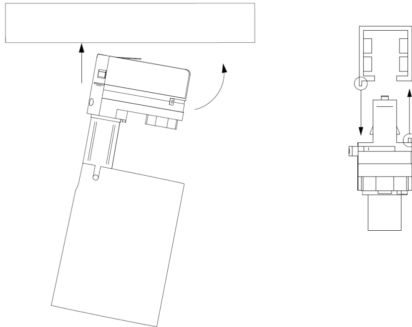
Anschluss an eine GLOBAL Trac Pro / Eutrac-Lichtschiene (Lichtschienensystem mit drei Schaltkreisen)
